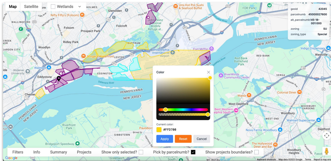
Инструмент “Палитра”
